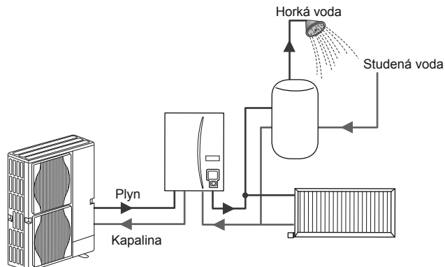
Schéma systému hydroboxu
